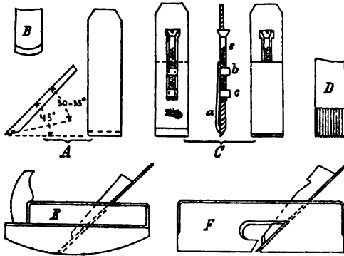
Č. 1726. Hoblíky truhlářské.
